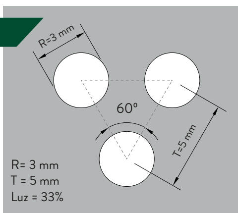
Dimensiones de perforación estándar
